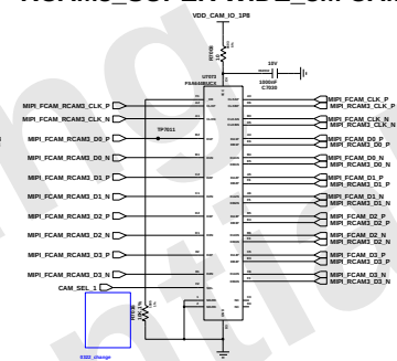
MIPI SWITCH (FCAM,RCAM3)
