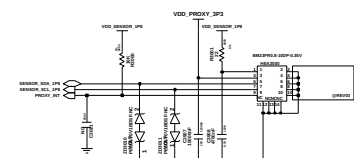
Proxy +RGB Sensor
