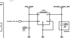
RCAM2 LDO
